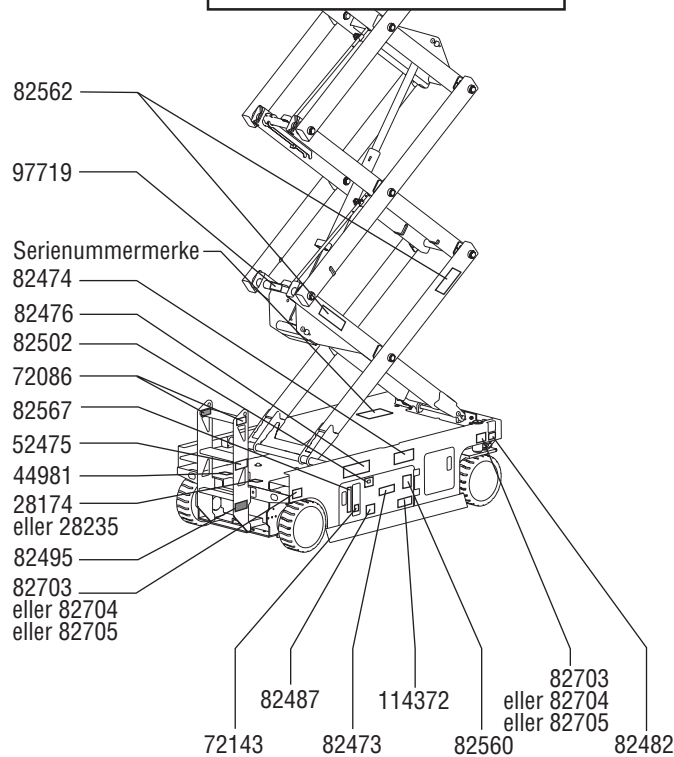
Bakkekontrollens side
