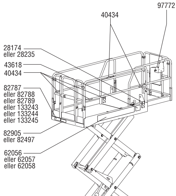
Bakkekontrollens side
