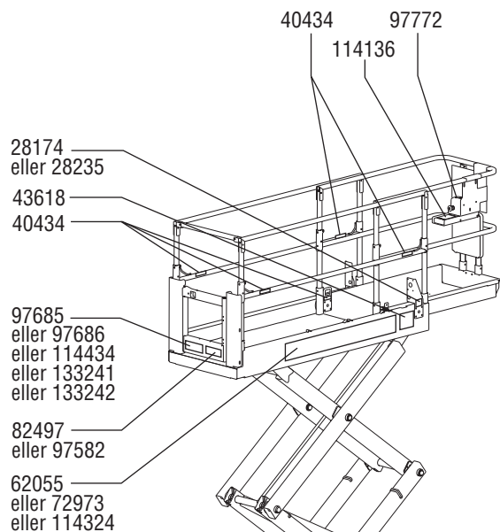
Bakkekontrollens side
