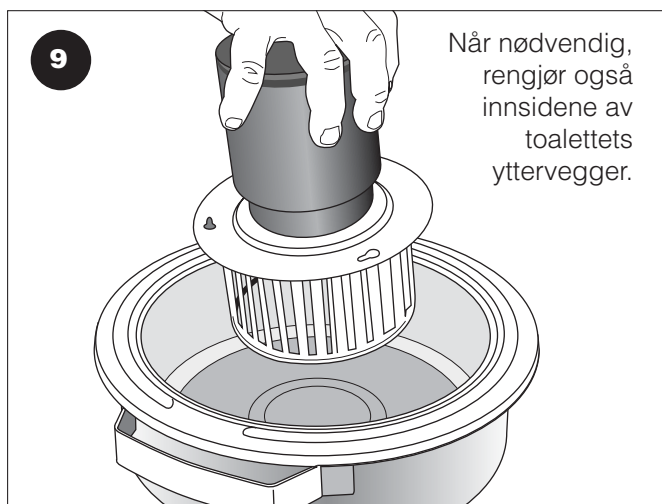
9 Senk viftehjulet ned i karet. Pass på at det ikke kommer vann opp i motordelen.
